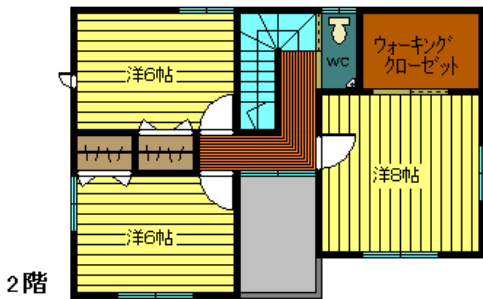
《間取り》
