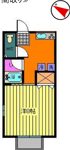
《間取り》
